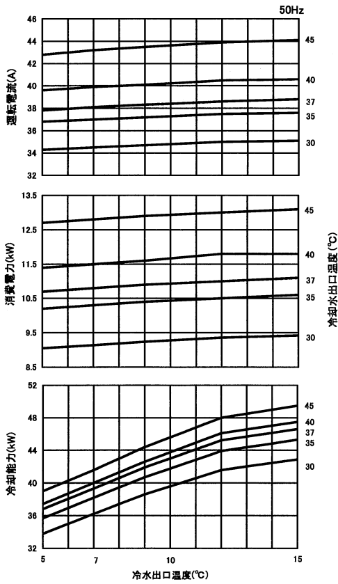
RUW-P 4501
