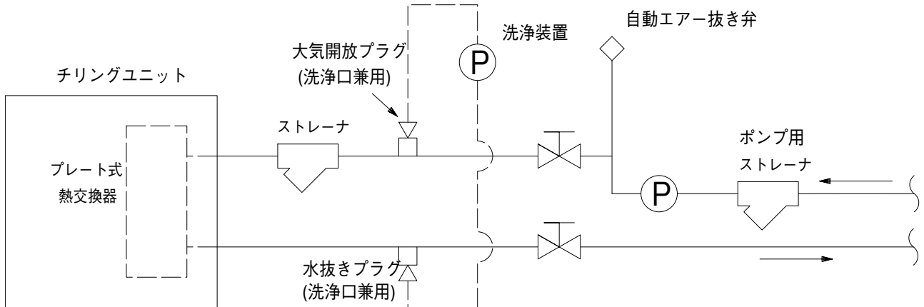
配管施行例
