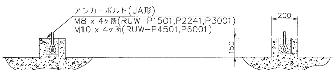
基礎コンクリート施工図(参考)
