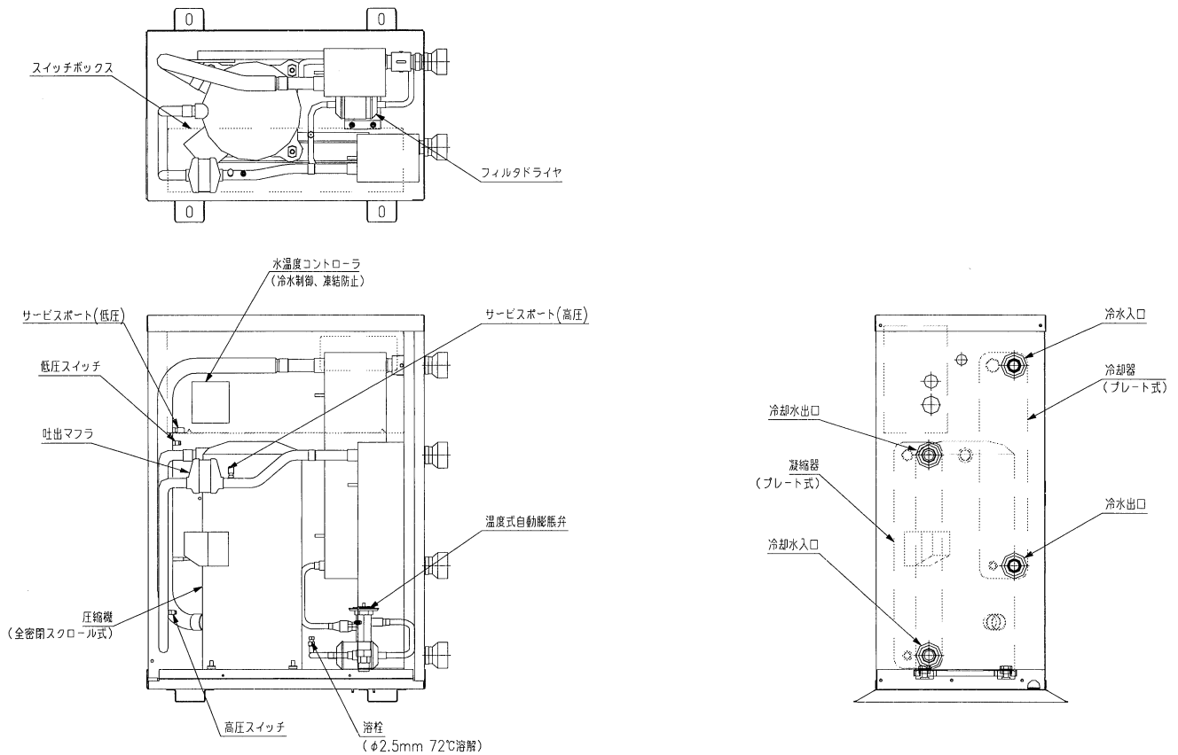
R U W - P 2 2 4 1, P 3 0 0 1
