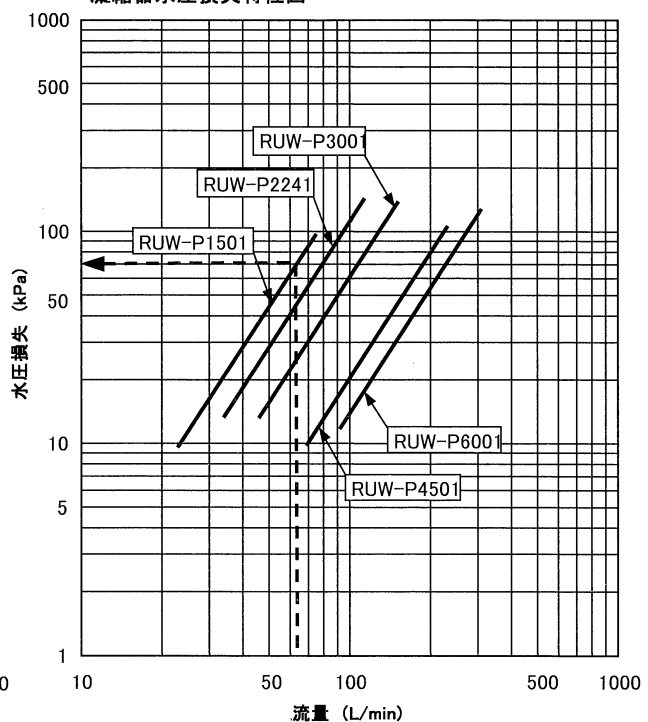
凝縮器水圧損失特性図
