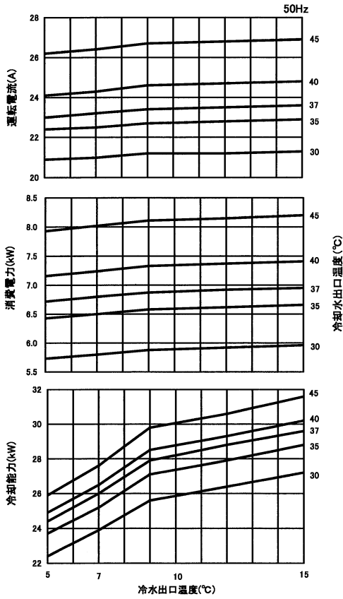
RUW-P 3001
