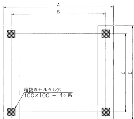
↓ 機器正面側
