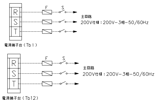
RUA-SFA30003HW～50003HW-A/B
