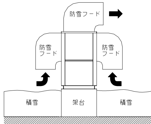
積雪地域における据付
