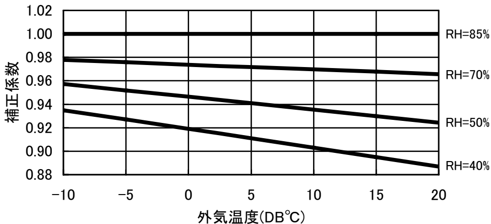
加熱能力相対湿度補正線図
