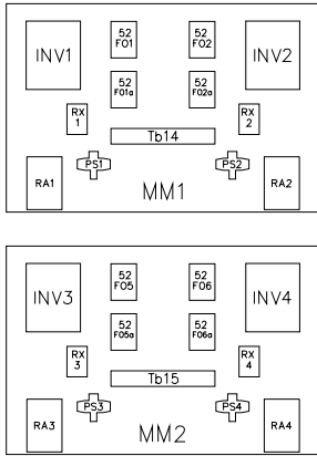
モータスタックボックス
