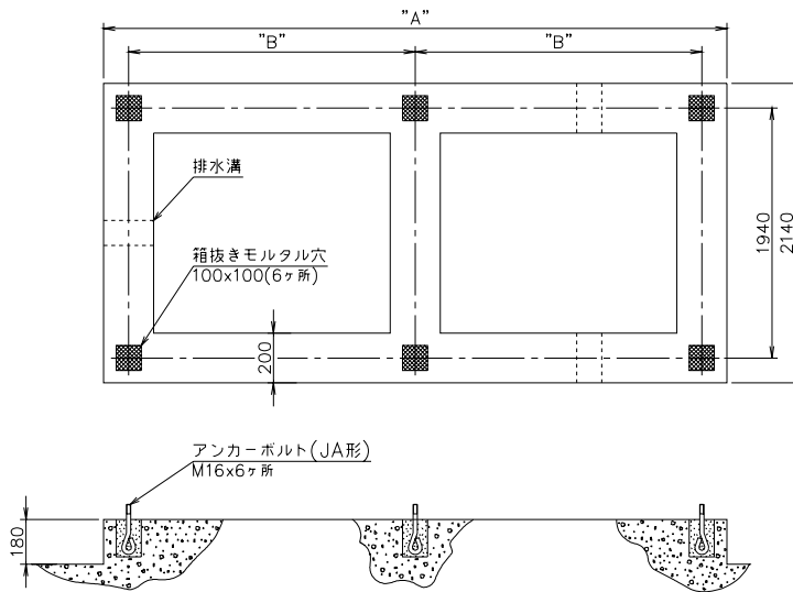
基礎コンクリート施工図
