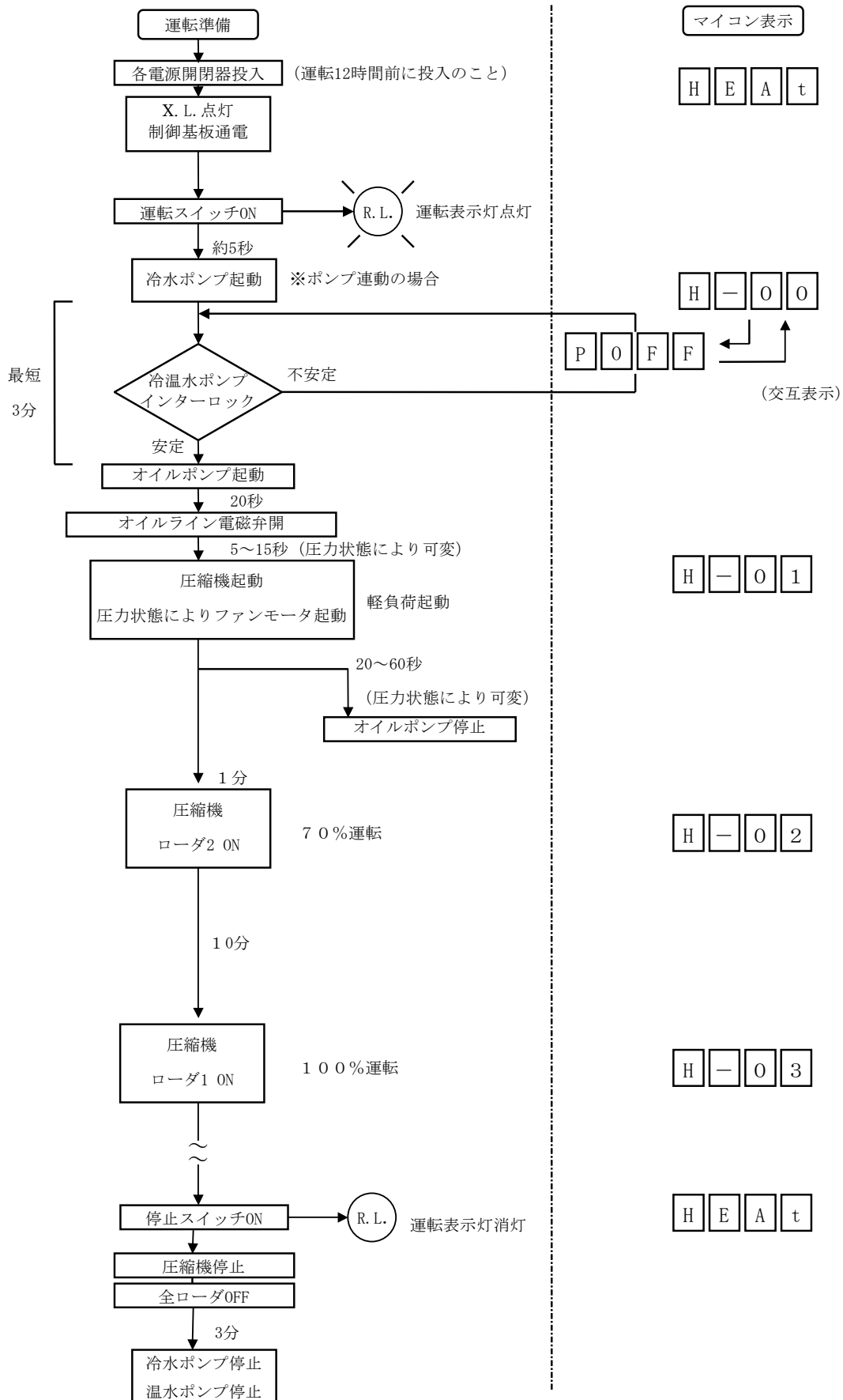
RUA-SFA150003HW～25003HW ユニット起動/停止フローチャート
