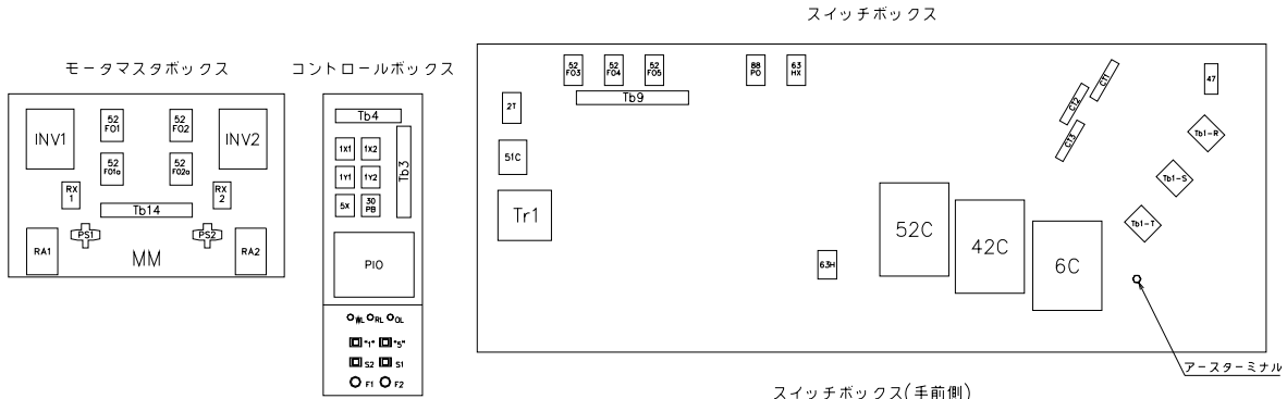
機器配置図
