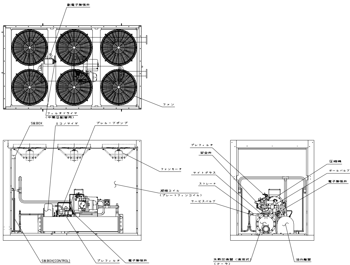
RUA-SB30005-B, SB31505-A
