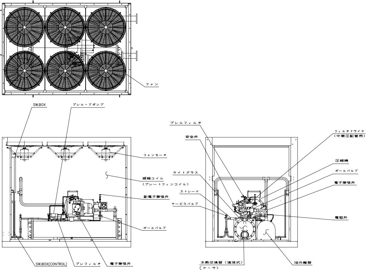
RUA-SB23605-A/B、SB30005-A
