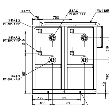
背面図
