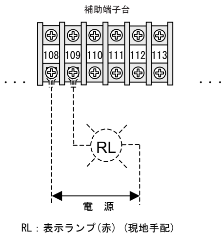
運転表示回路の結線
