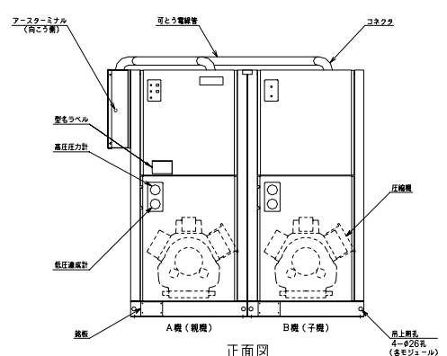
正面図
