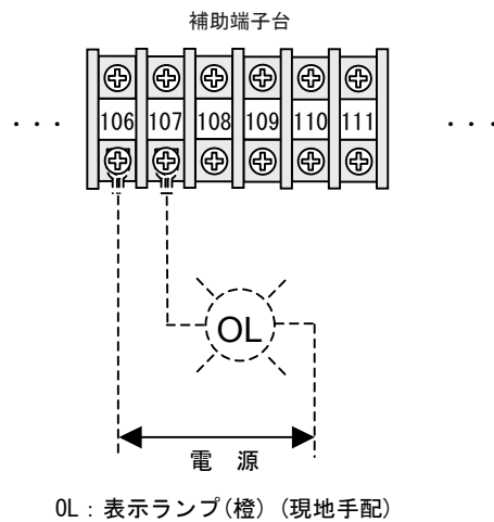
故障表示回路の結線
