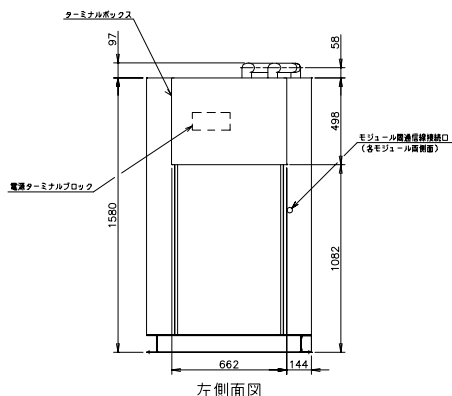
左側面図
