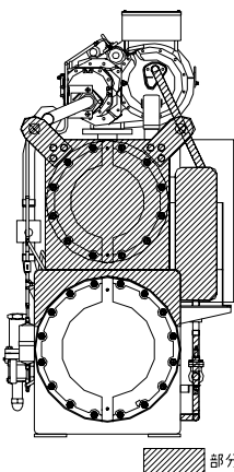
■部分は保冷施工部分を示します
