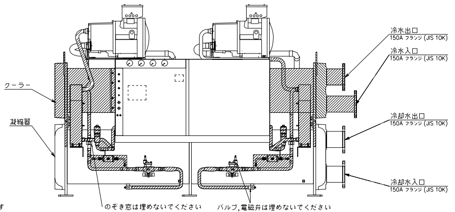
■部分は保冷施工部分を示します
