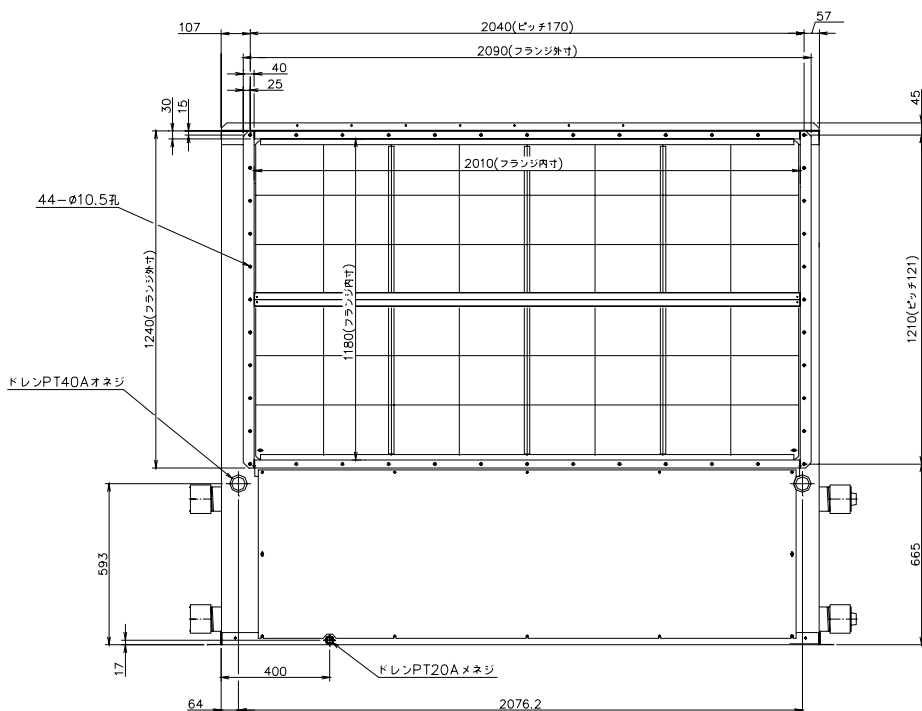
背面図
