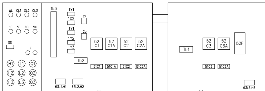
スイッチボックス機器配置図
