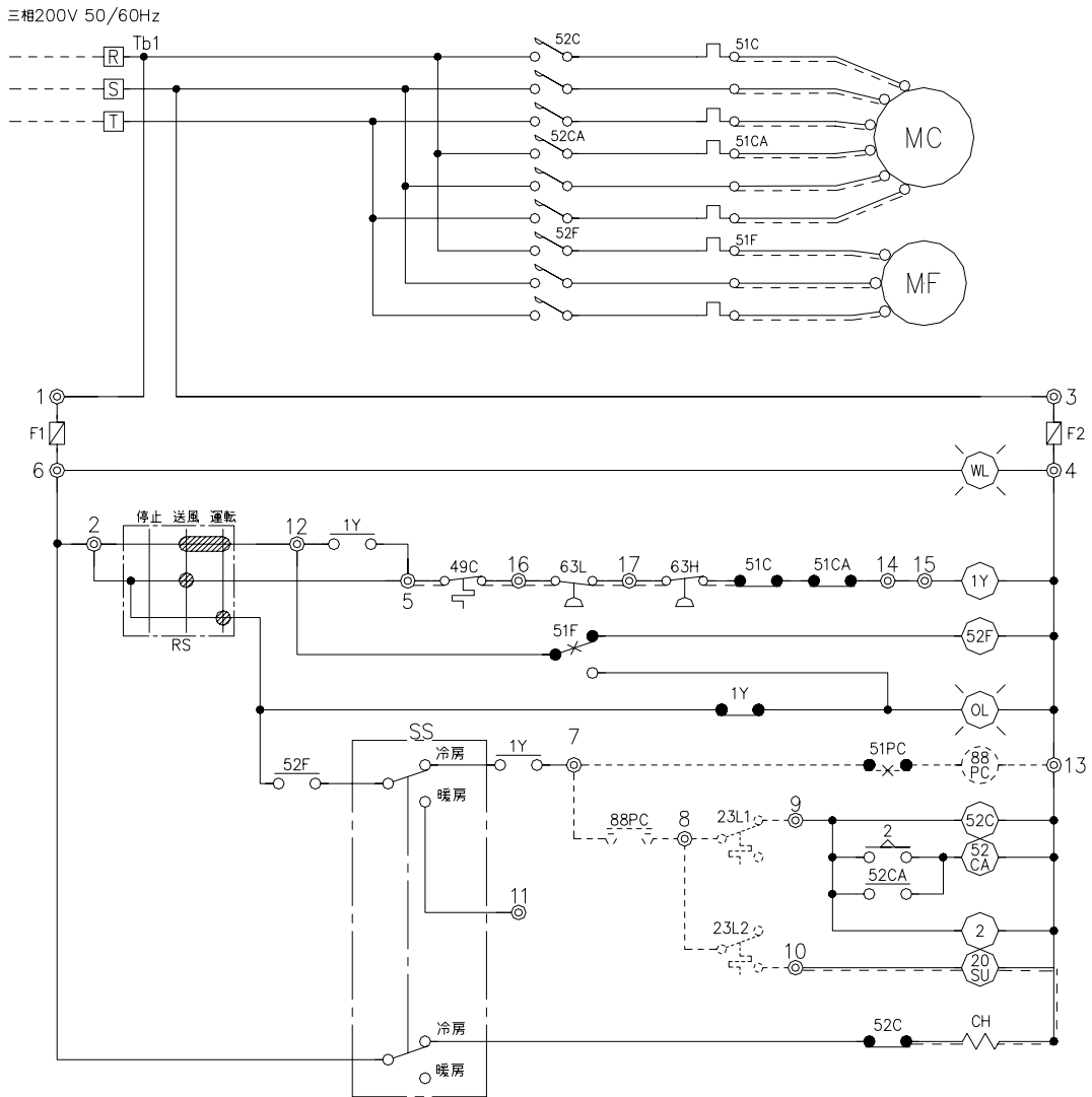
コントロールパネル
