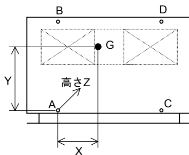
概略図 b
