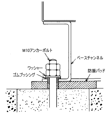
基礎ボルト取付施工図 (参考: 矢視D)
