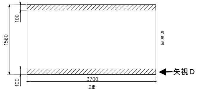
防振パッド取付位置
