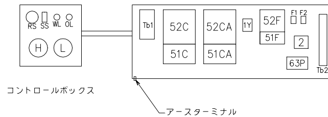
スイッチボックス、コントロールパネル機器配置図
