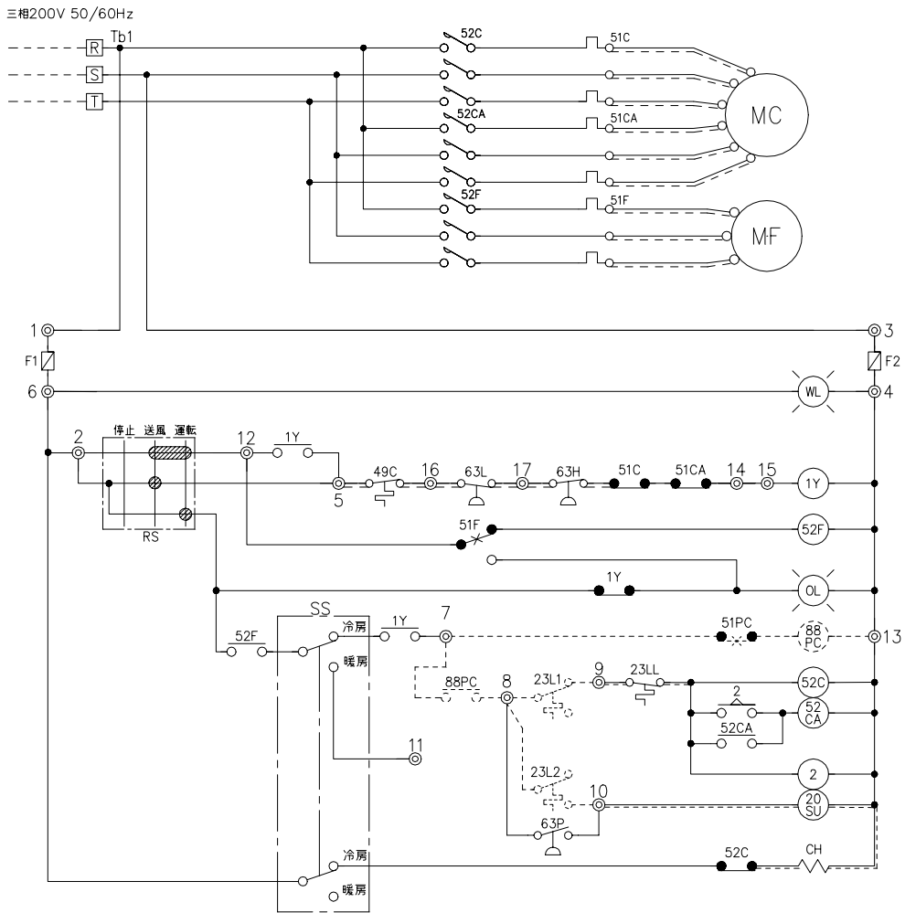
コントロールパネル
