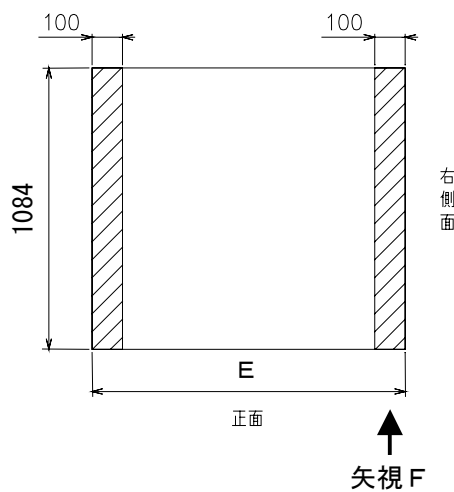
防振パッド取付位置
