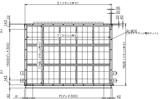
背面図
