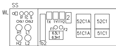
スイッチボックス、コントロールパネル機器配置図
