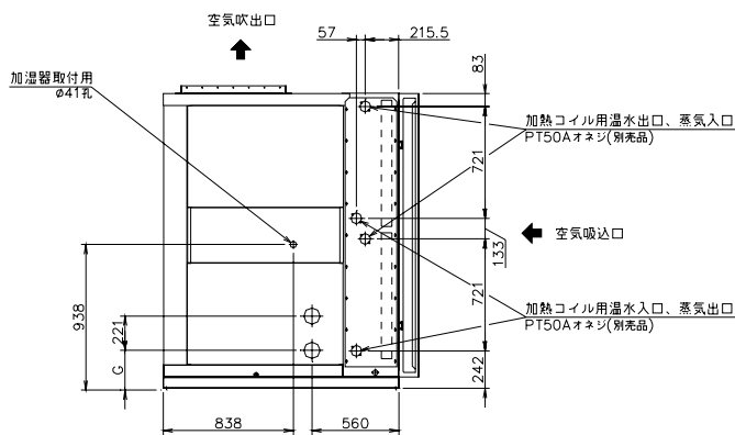
右側面図
