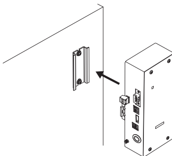
Wandhalterung B
