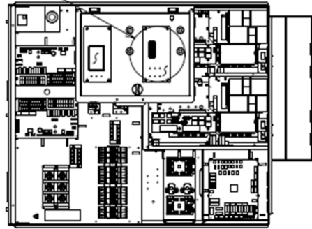
機器配置図
