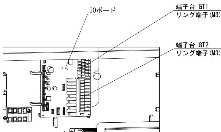
図2 詳細図
