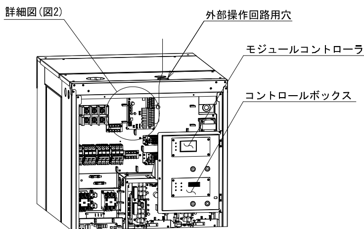
図1 熱源機外部配線接続例
