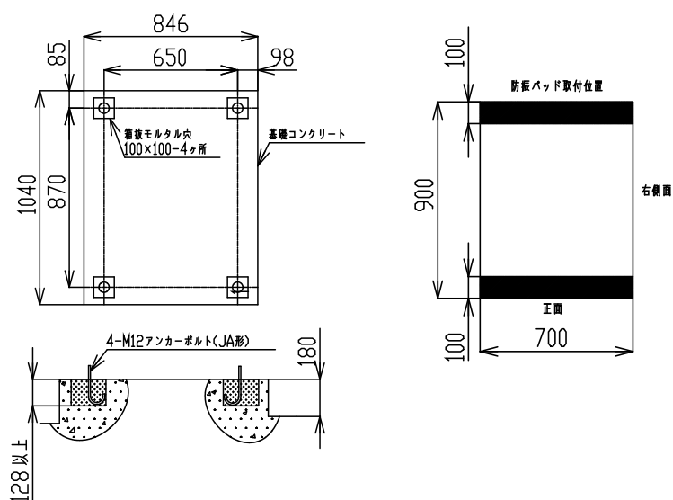
据付基礎図
