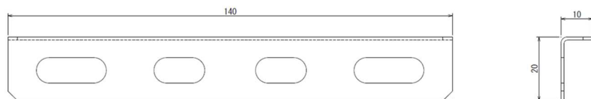
連結金具
