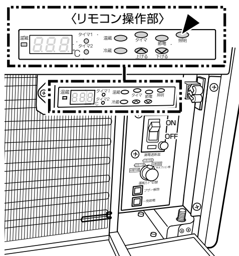
(機械室カバーを開けた状態)
