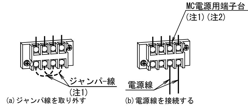
図3 ジャンパ線配線例
