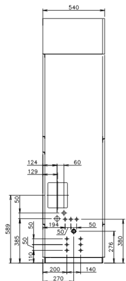
右側面図
