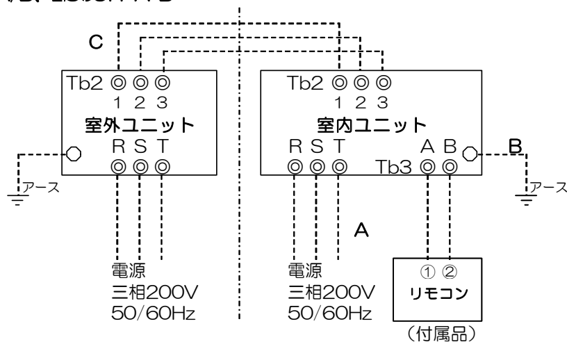
図-8 配線結線図
