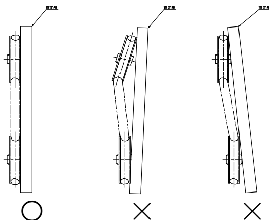
図-6 プーリの芯出し
