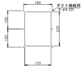
外気取入ダクト接続口(右側面図)
