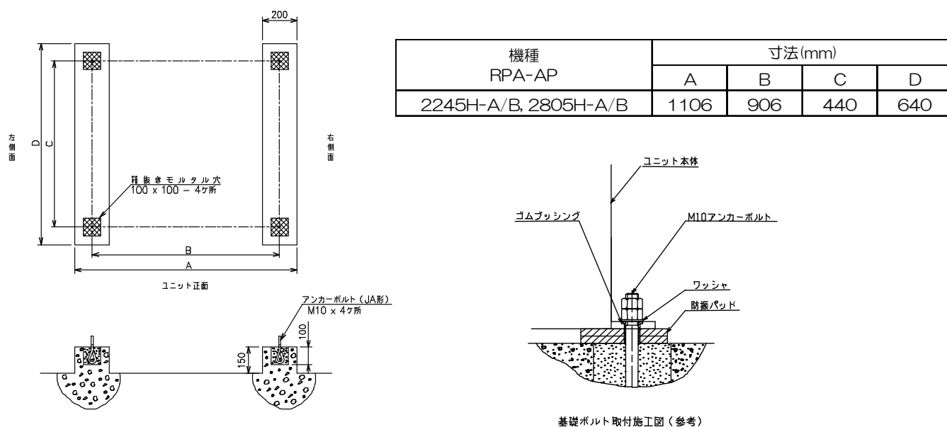
図-3 据付基礎施工図(参考)
