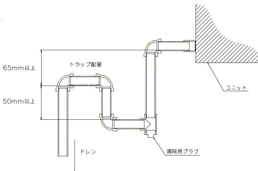
図-5 ドレン配管
