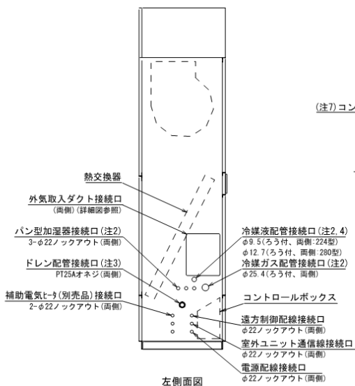
左側面図
