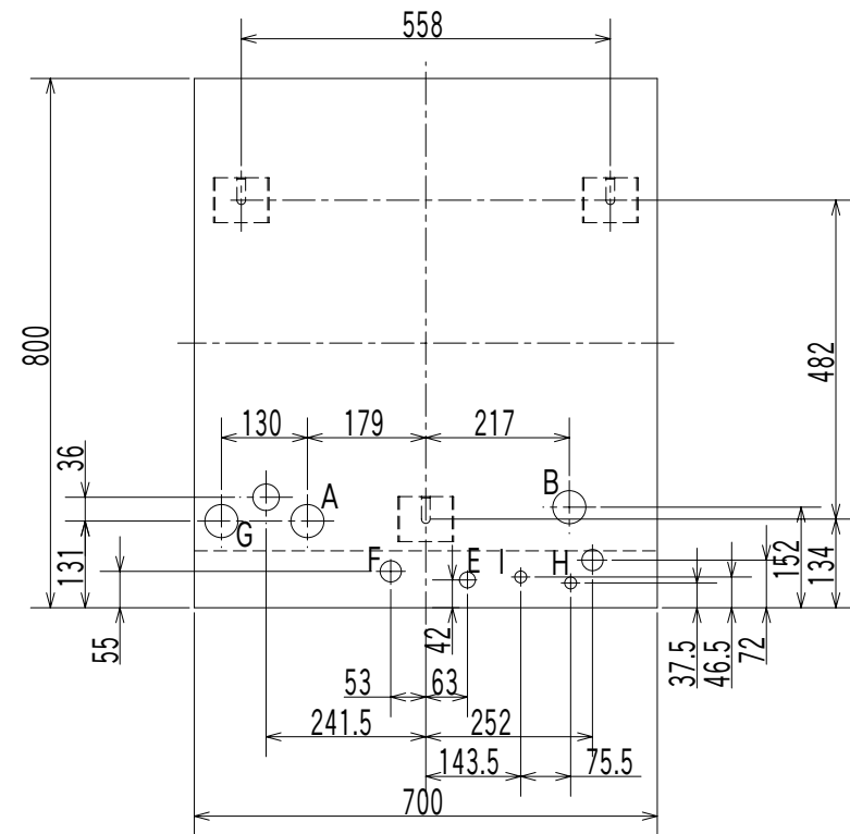
接続口位置図 (製品上面図) アンカーボルト位置図
