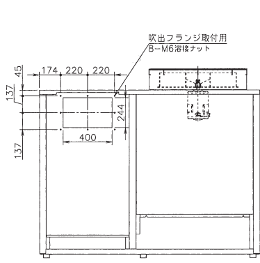
背面図
