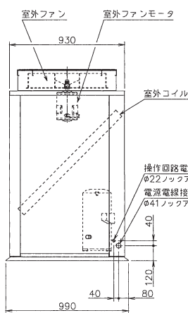
左側面図
