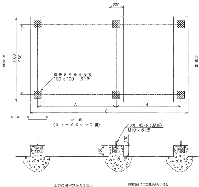
基礎コンクリート施工図（参考）
