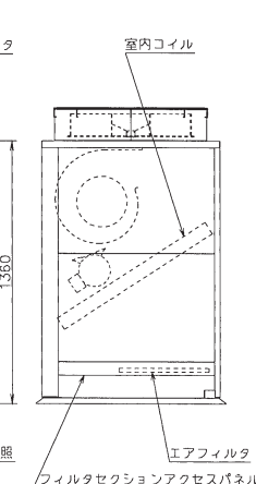
右側面図
