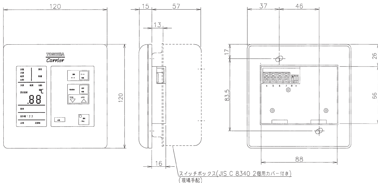
外形寸法図
