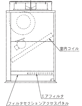
右側面図
